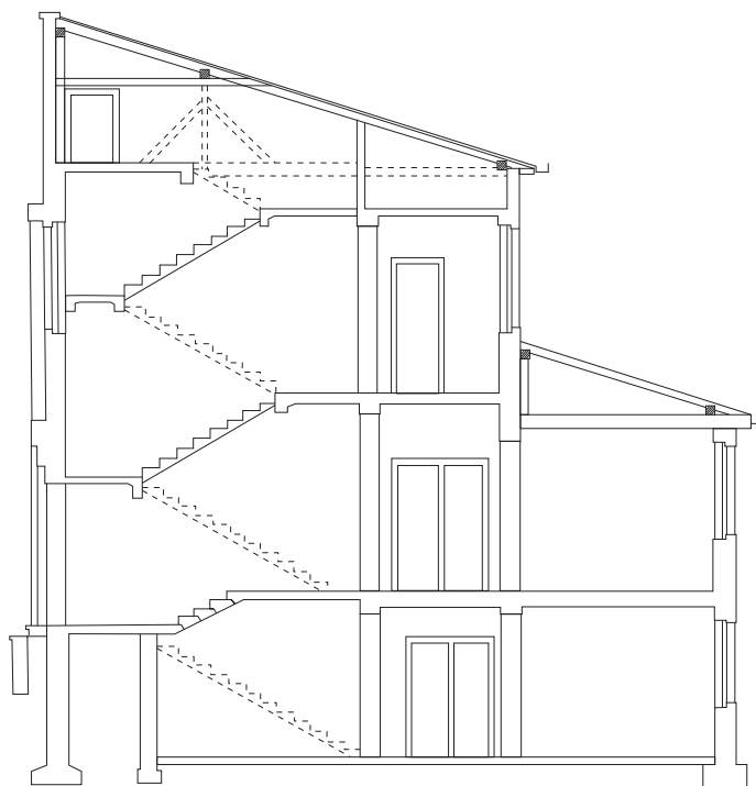
Слика 54: План попречног пресека соколског дома
