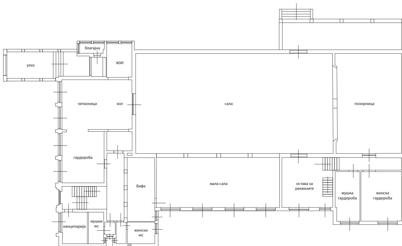
Слика 53: План основе приземља соколског дома
